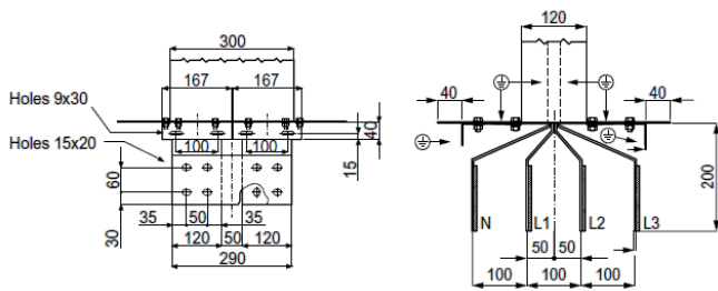
Cu 2500A
