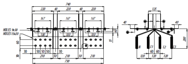
Al 5000A
