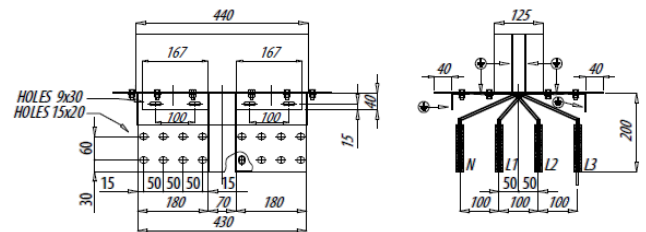
Cu 4000A
