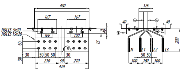
Cu 5000A
