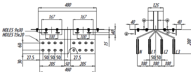
Al 4000A
