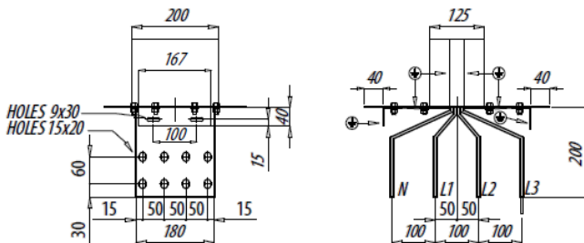
Al 1600A
