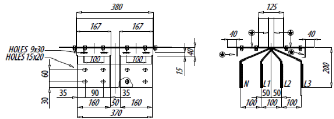
Cu 3200A
