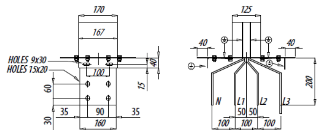
Cu 1600A-2000A
