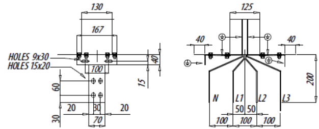
Cu 800A
