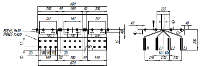
Cu 6300A
